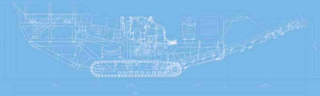
Схема MR 170 Z в рабочем положении
