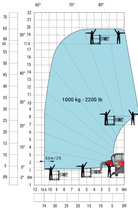
Вращение башни при опущенных аутригерах с платформой 1000 кг
